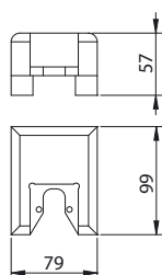
Base per applicazione verticale
