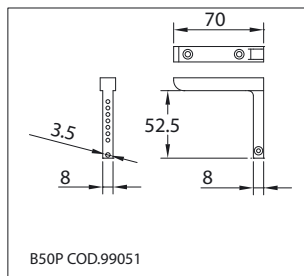
Becca in dotazione Jaw standard
