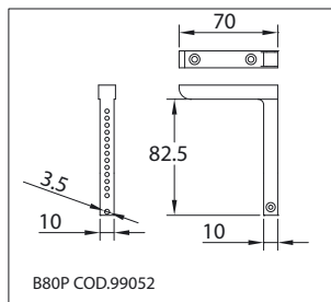
Becca opzionale Optional jaw
