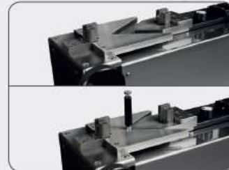
Control of diameter and 3 point micrometer Controllo diametri e micrometri a 3 punti
